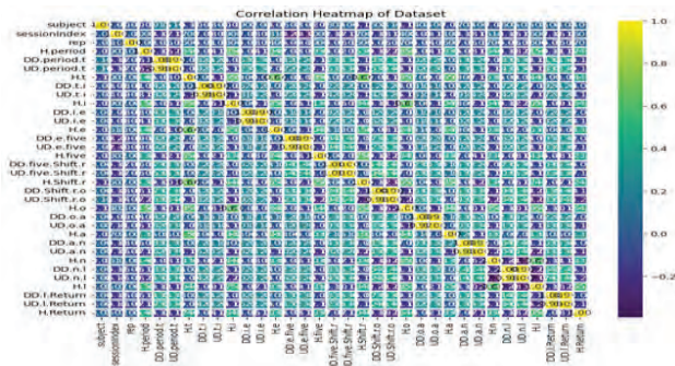
Fig. 2 : Dataset Heatmap
