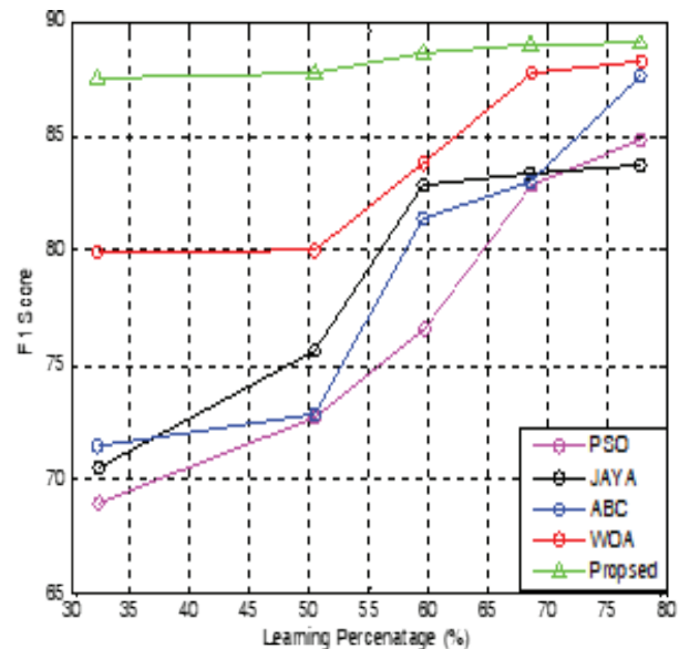
Fig. 5: F1 Score
