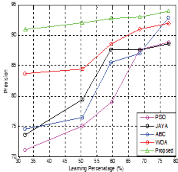
Fig. 6: Precision
