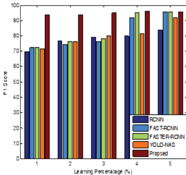
Fig. 9: F1 Score
