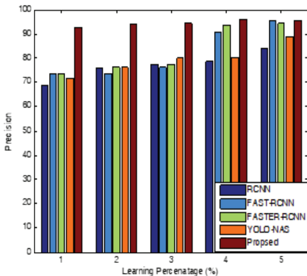
Fig. 10: Precision
